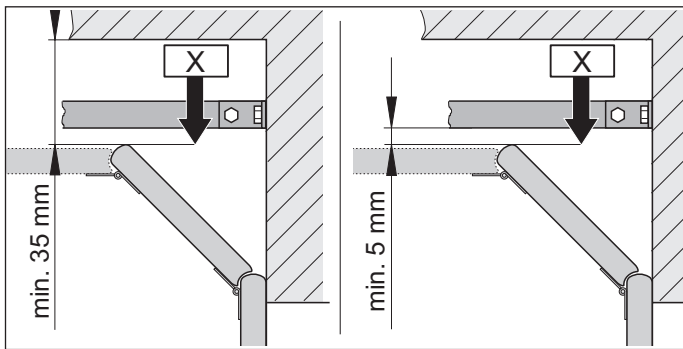
Abb. 1.2 Torhöchstlaufpunkt Sektionaltore
