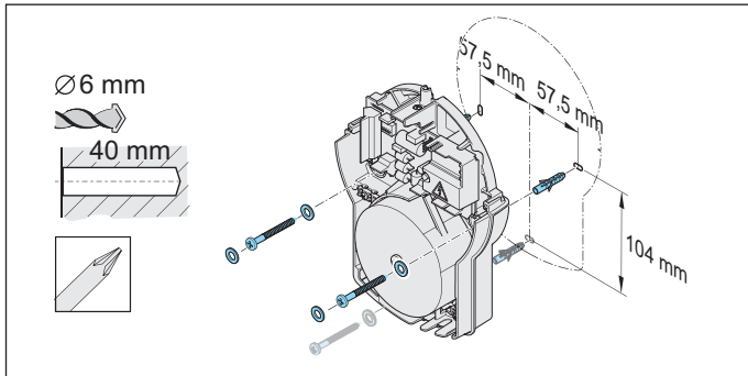
Abb. 4: Montagebeispiel
