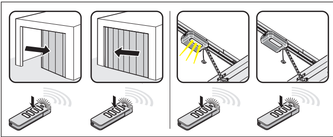
Impulsfolge für: Teilöffnung: DIP-Schalter 2 auf „ON“ Beleuchtungsfunktion: DIP-Schalter 2 auf „OFF“
