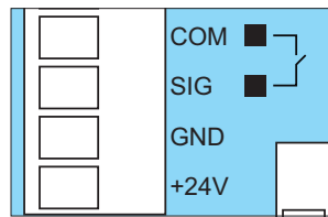
Abb. 2 Anschlussklemme für eine 4-Draht-Lichtschanke
