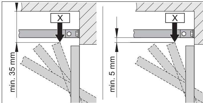
Bild 1.1: för portens högsta löppunkt för utåtgående och inåtgående vipport
