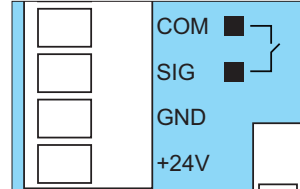
Anslutningsklämma för 4-ledad fotocell
