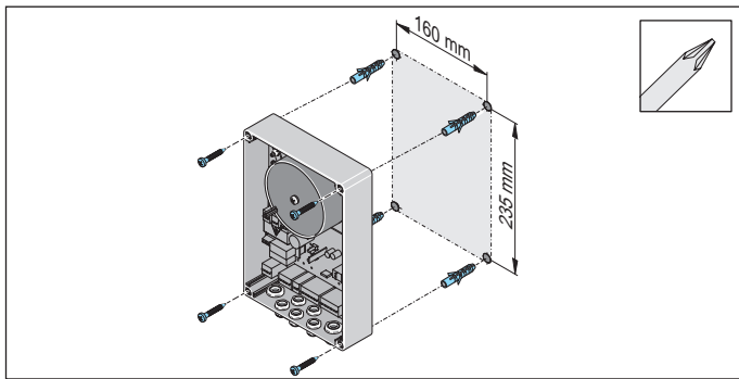
Afb. 3 Montagevoorbeeld
