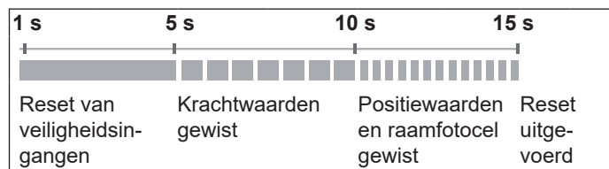
Afb. Overzicht van volgorde in tijd van de status-LED op de pla-fondbesturing bij het indrukken van de groene resetknop
