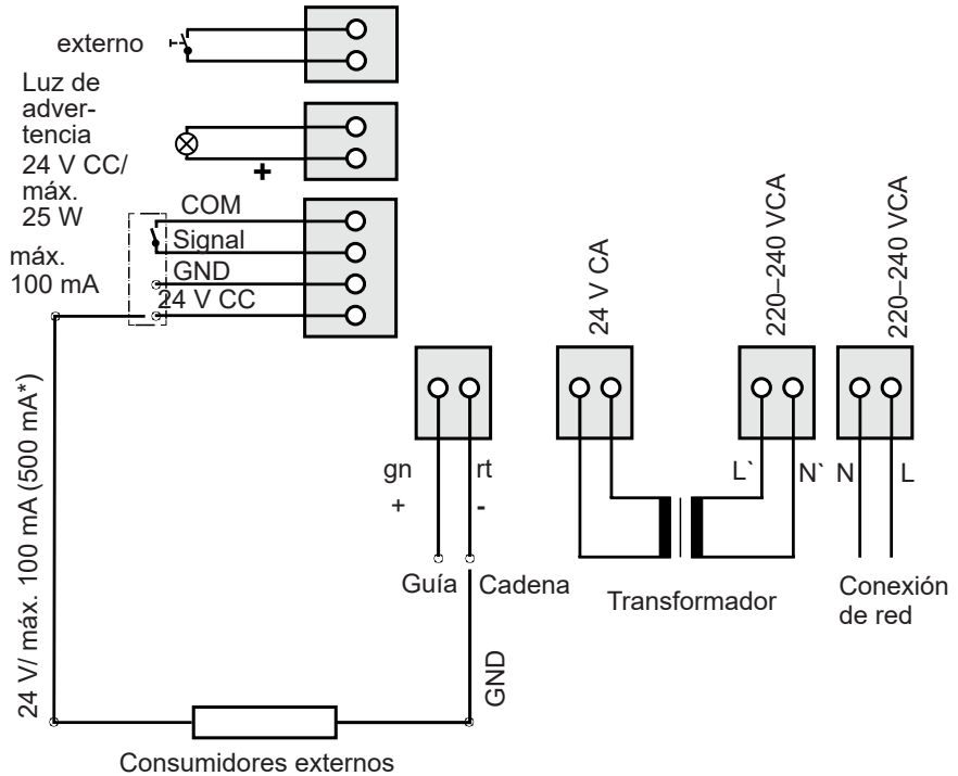
Fig. Esquema de conexiones del cuadro de techo
