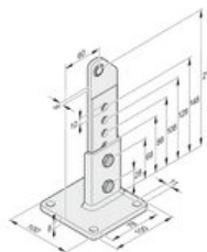
Ferrure de poteau à rotule 60/210 G
