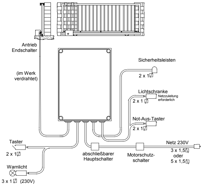
Bild 14 Installationsplan
